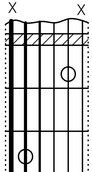
C sus2
