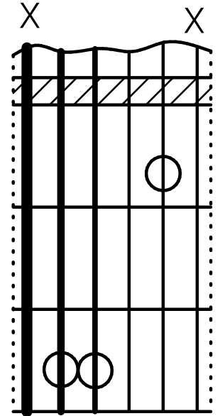
C sus4
