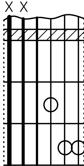
D sus
