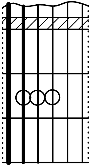
G sus4
