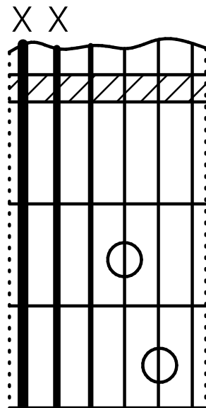
D sus2
