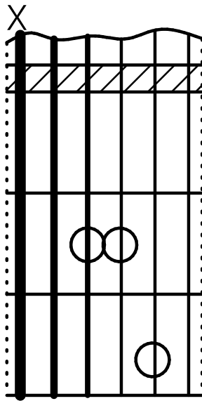
A sus
